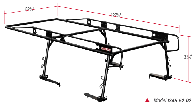
▲ Model 1345-52-02
