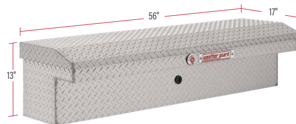
▲ Model 178-0-04
