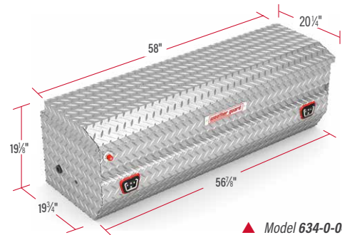
▲ Model 634-0-04
